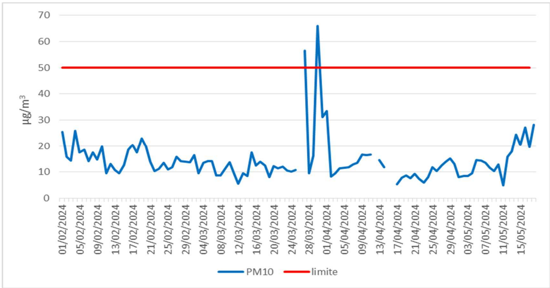
Figura 2a. Media giornaliera di PM10
