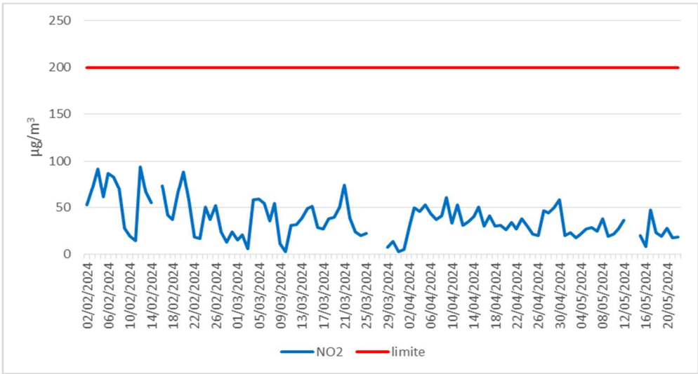
Figura 3b. NO 2 : massimo giornaliero della media oraria
