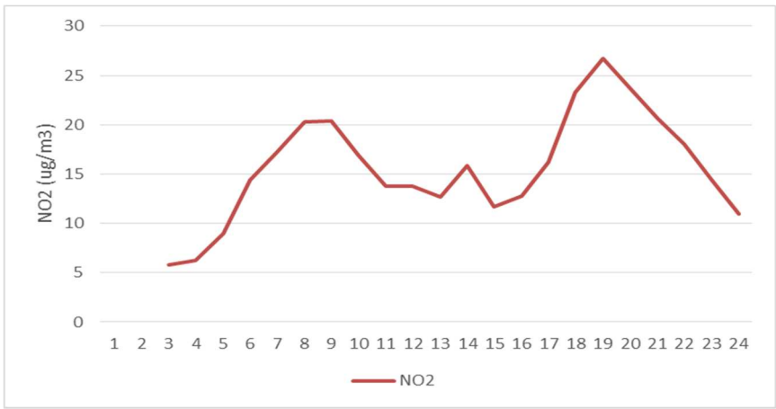
Figura 3c. NO 2 : giorno tipo
